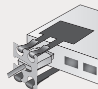
③ 面ファスナーを折り返し、しっかり合わせる。 Fold back the fastener belts and tighten.
