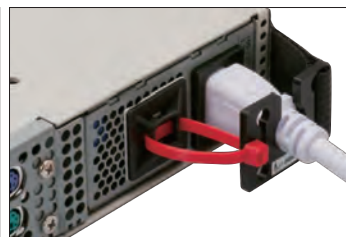
●市販のバンド利用 Commercial cable tie being used.
