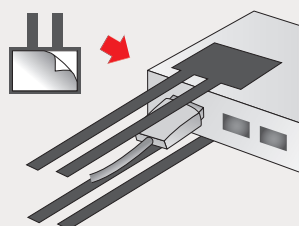
① 粘着付面ファスナーを機器に取り付けます。 Attach adhesive fastener to device.
